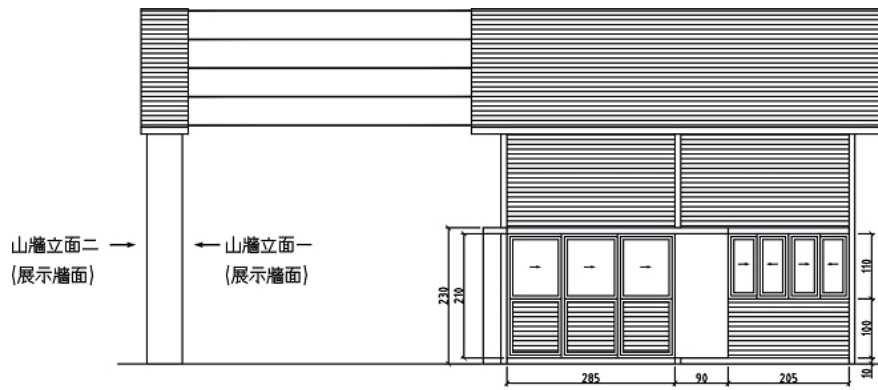
木屋東向立面修繕與假牆
