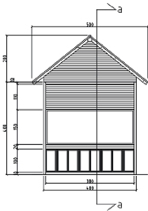
山牆立面一(展示牆面)
