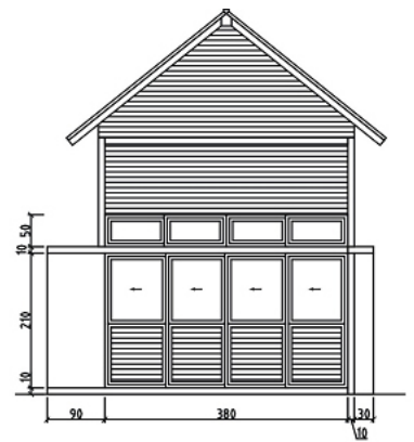
木屋南向立面修繕
