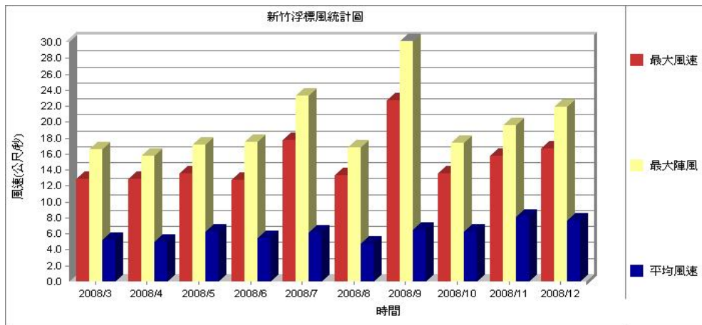
圖 6 新竹縣沿海風速風向統計圖（92 年度）
