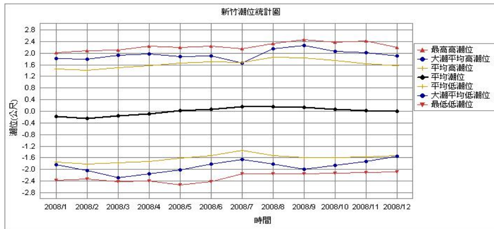
圖 4 新竹縣沿海潮汐圖 (97 年度)
