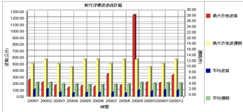
圖 7 新竹縣沿海波浪統計圖 (97 年度)
