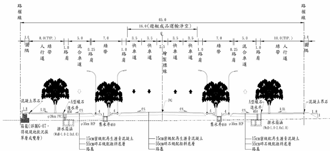
圖 2-10 道路施工標準斷面圖(0K+690~1K+843.081)
