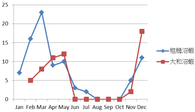
圖 2-3、老人溪測站之甲殼類數量月別變化圖
