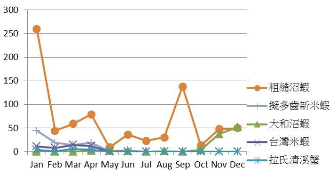
圖 2-5、民權橋測站之甲殼類數量月別變化圖
