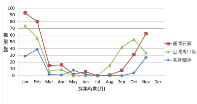
圖 1-7、西安吊橋測站主要魚種族群數量月別變化圖
