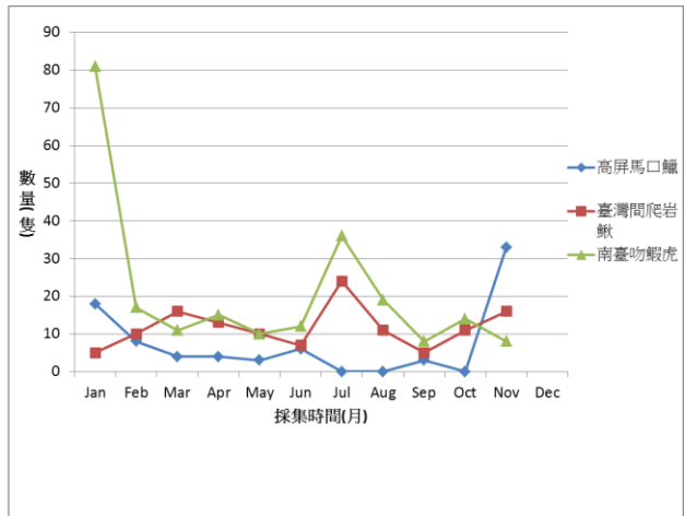
圖 1-6、民權橋測站主要魚種族群數量月別變化圖
