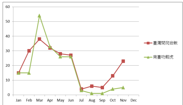
圖 1-3、長春谷測站主要魚種族群數量月別變化圖
