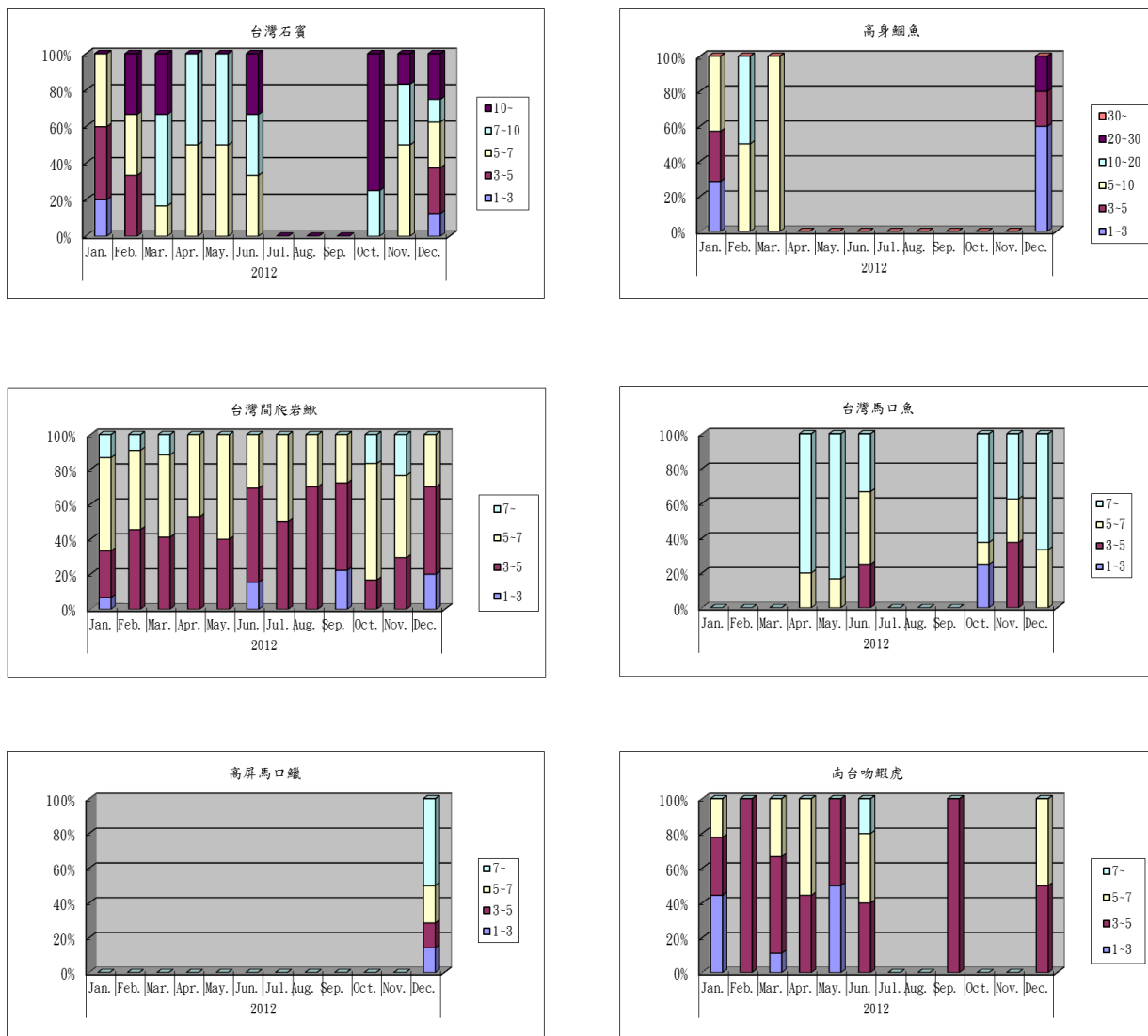
圖 1-17、一溪吊橋測站主要優勢魚種體長組成及相對數量圖
