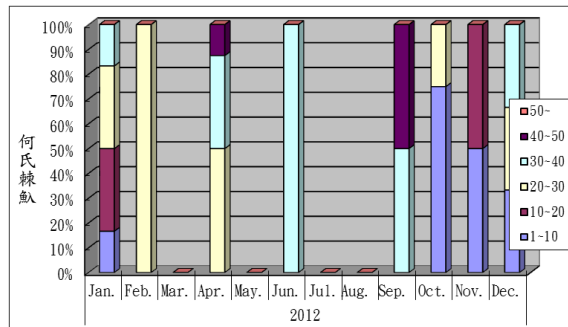
圖 1-20a、小林測站主要優勢魚種體長組成及相對數量圖
