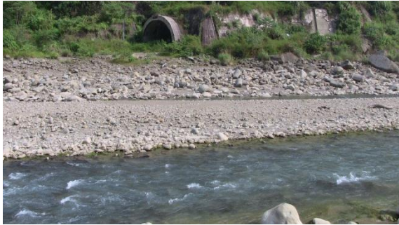
圖 8. 贏橋測站
